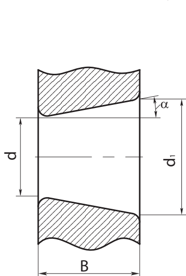
Рис. 9. Номинальное коническое отверстие
