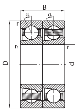
Схема комплектования «тандем» замок на внутреннем кольце
